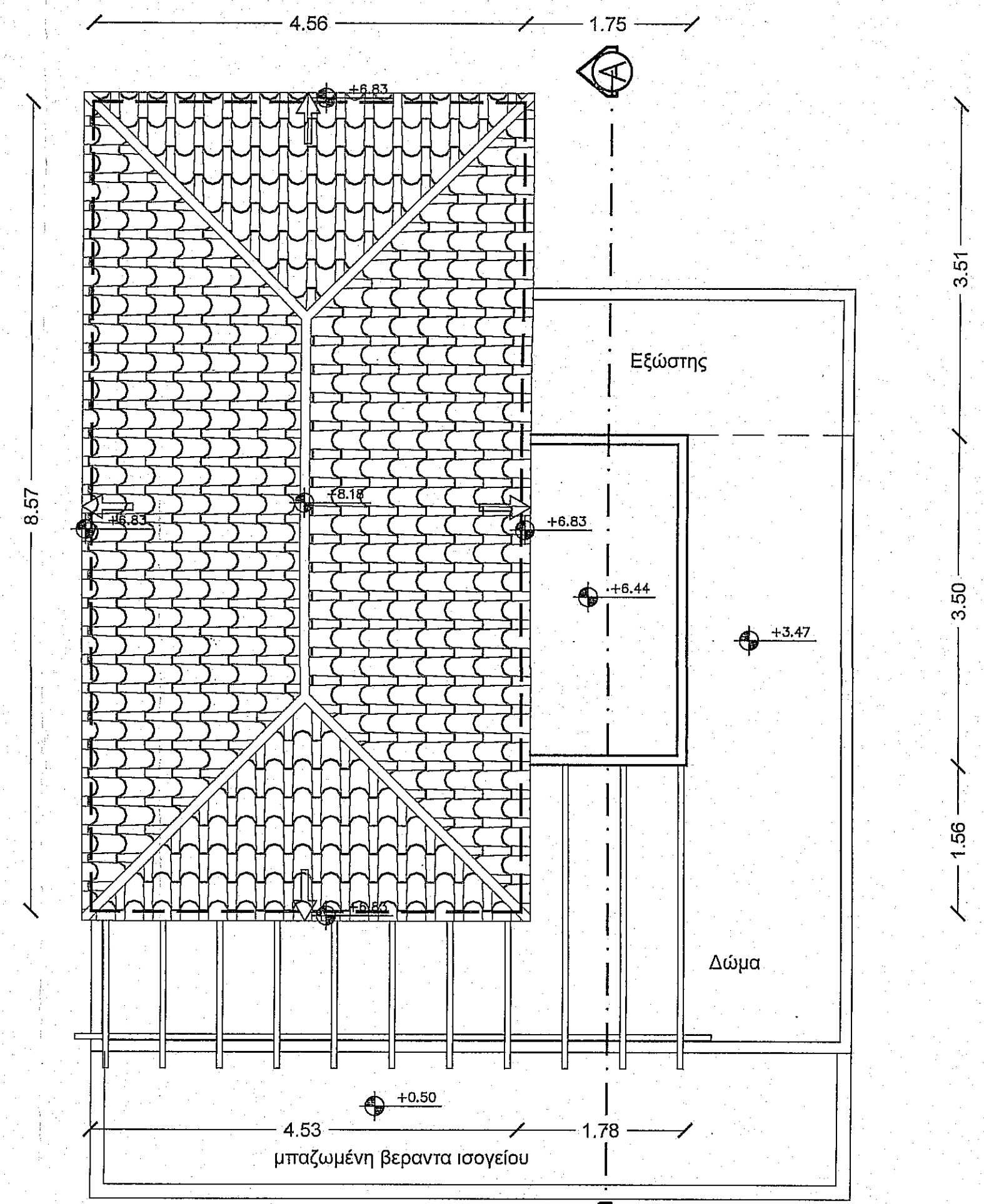
ΚΑΤΟΨΗ ΔΩΜΑΤΟΣ
