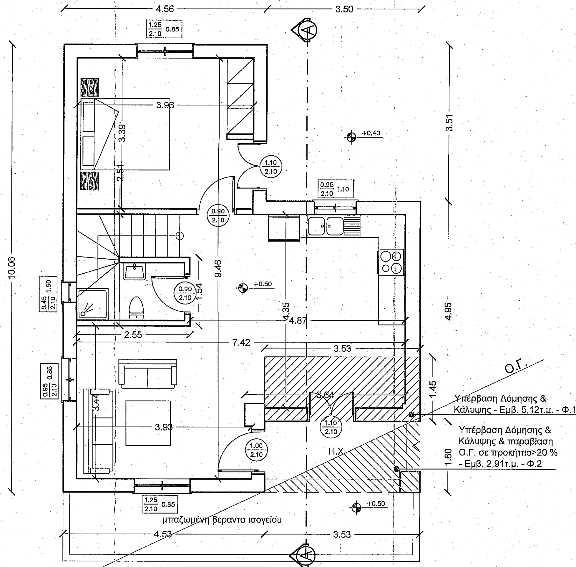
ΚΑΤΟΨΗ ΙΣΟΓΕΙΟΥ
