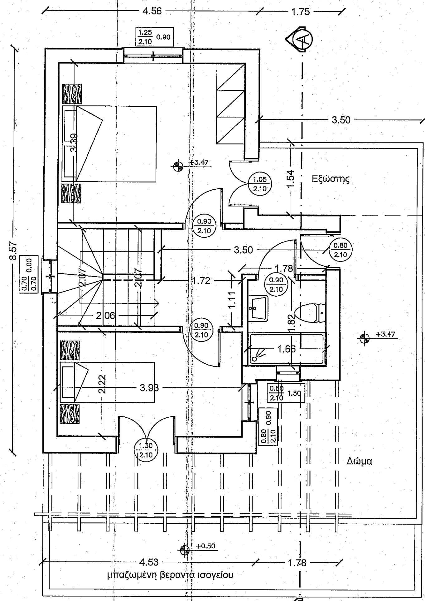
ΚΑΤΟΨΗ ΟΡΟΦΟΥ
