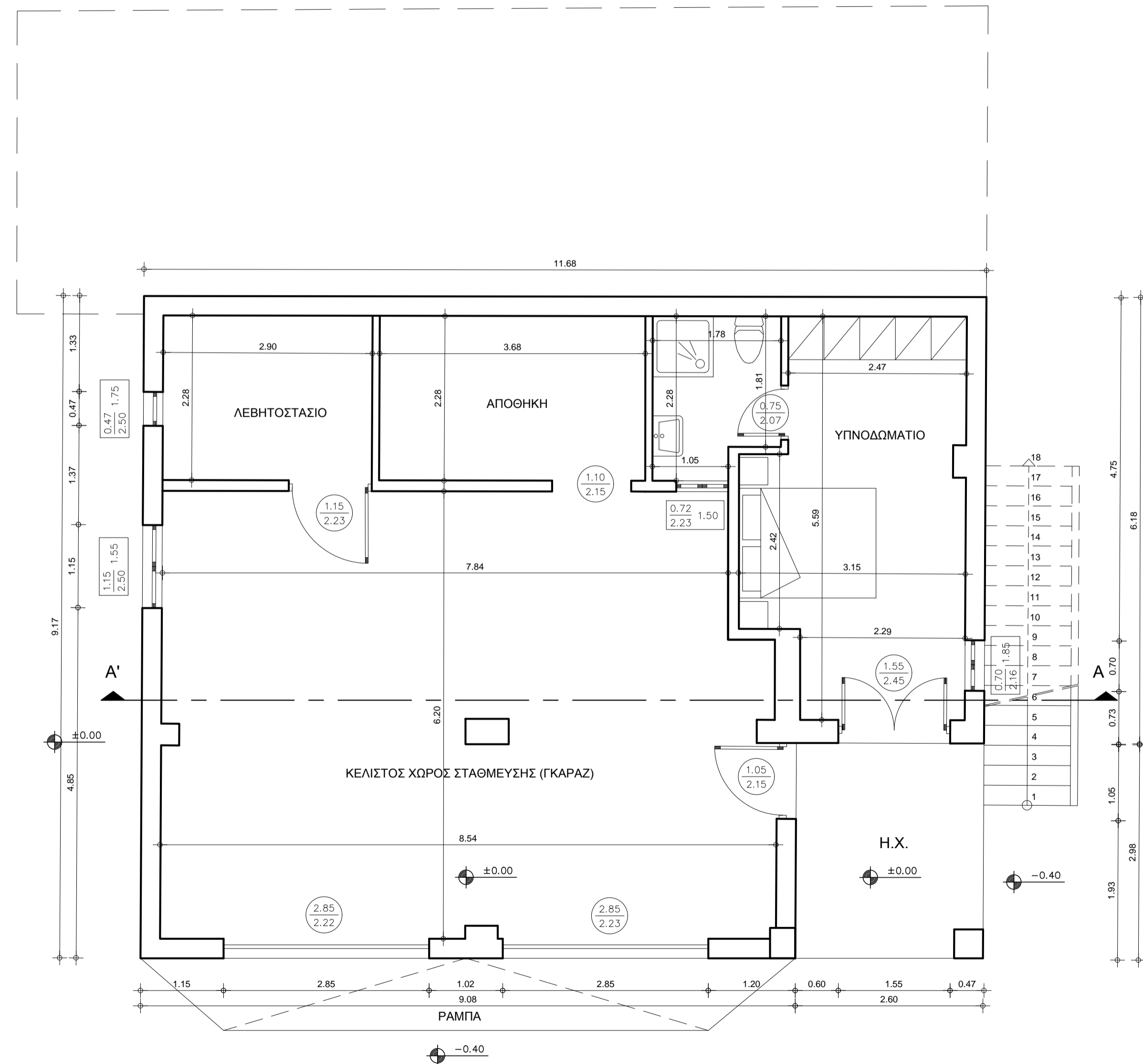
ΚΑΤΟΨΗ ΙΣΟΓΕΙΟΥ-ΥΠΟΓΕΙΟΥ (1η στάθμη)
