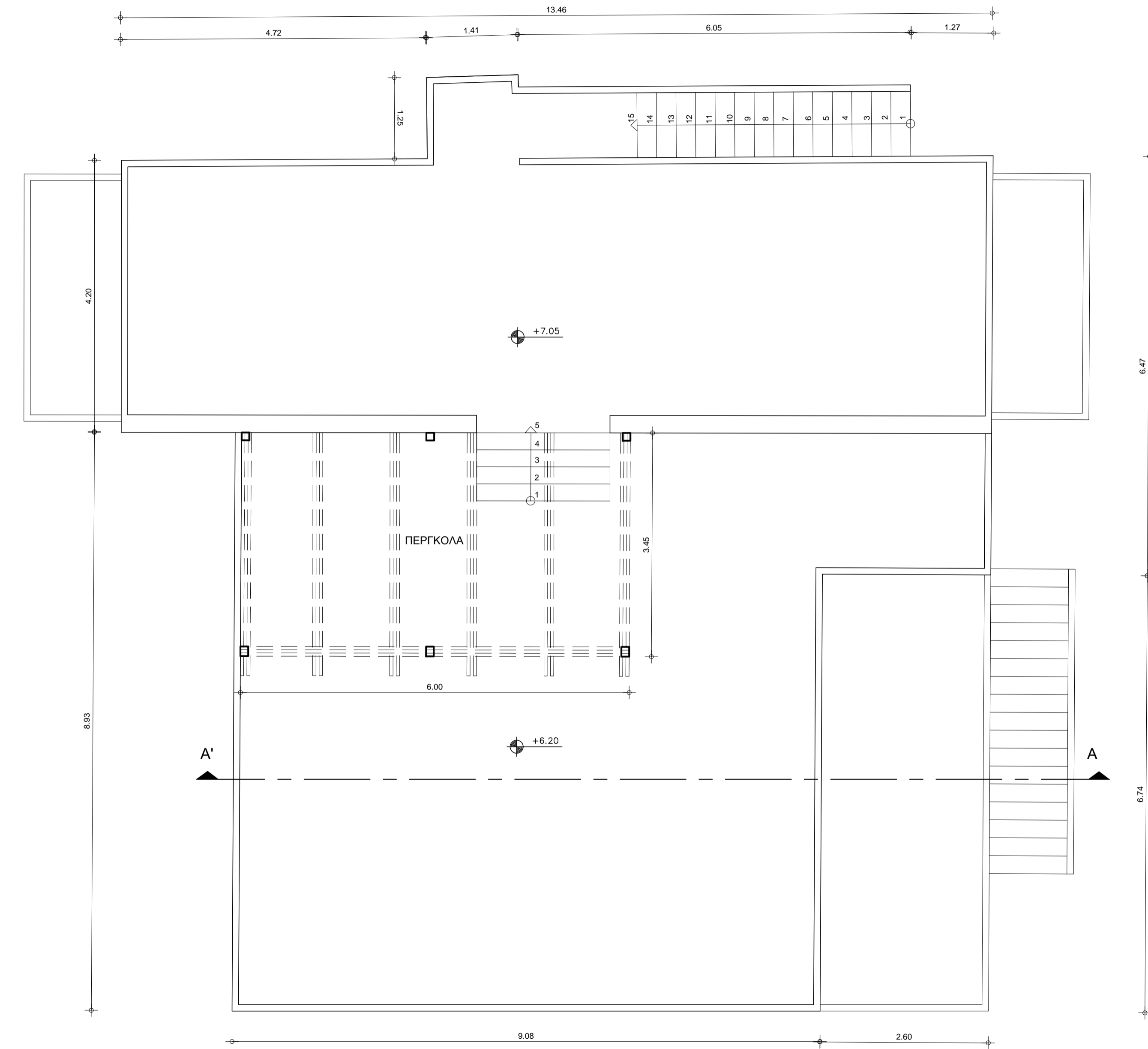
ΚΑΤΟΨΗ ΔΩΜΑΤΟΣ (3η στάθμη)
