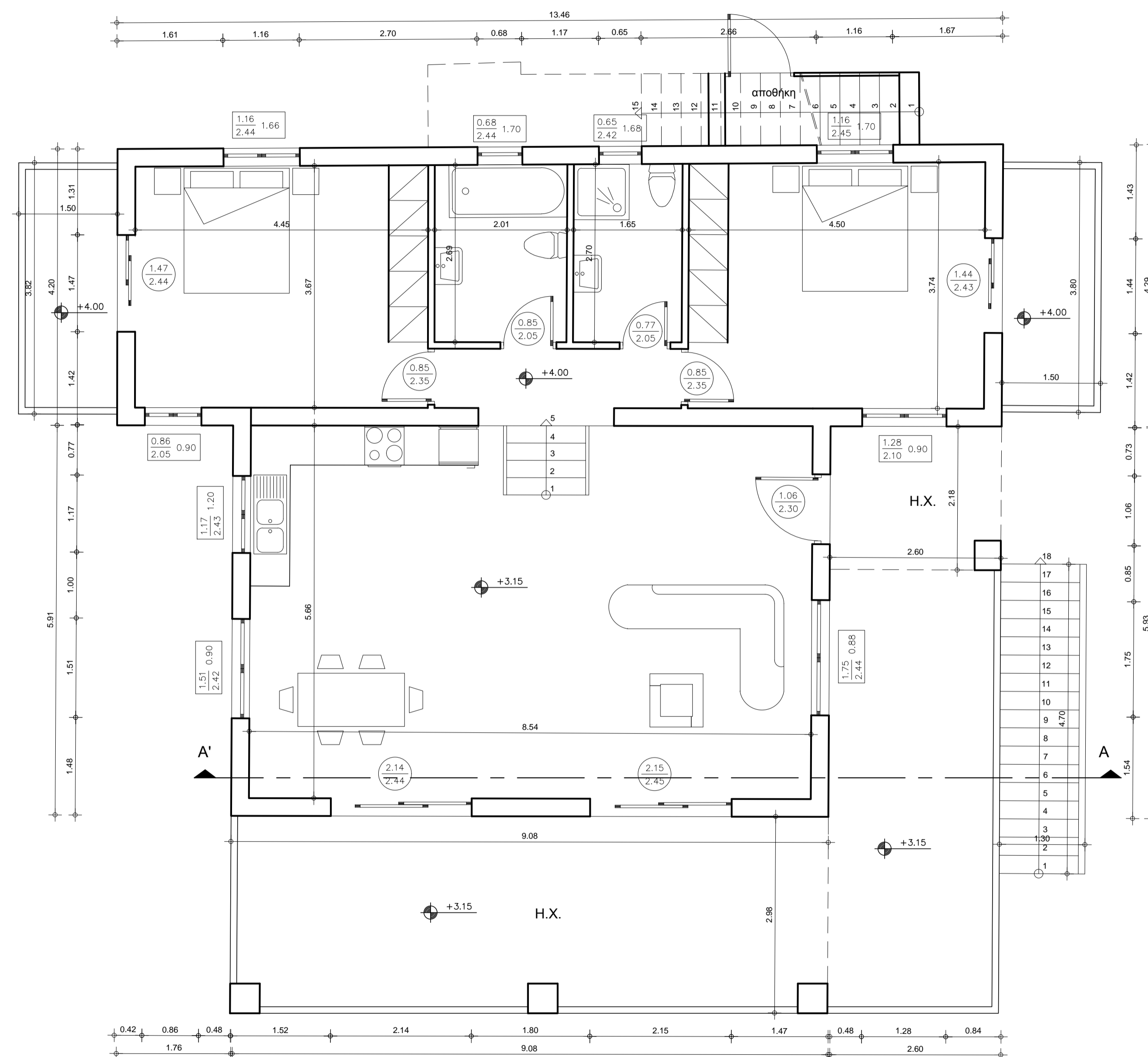
ΚΑΤΟΨΗ ΙΣΟΓΕΙΟΥ (2η στάθμη)
